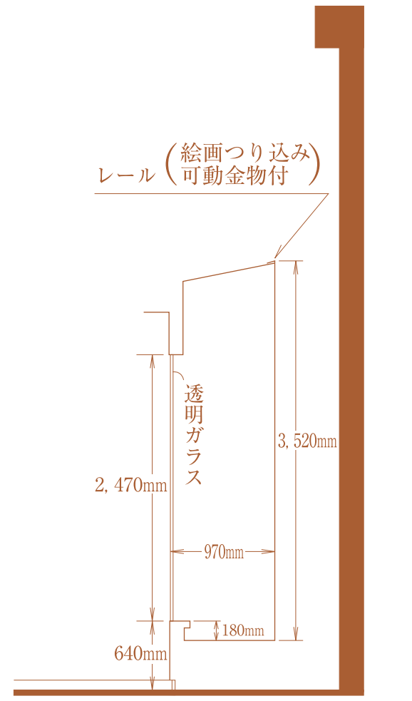
陳列ケース断面図 S 1/50
