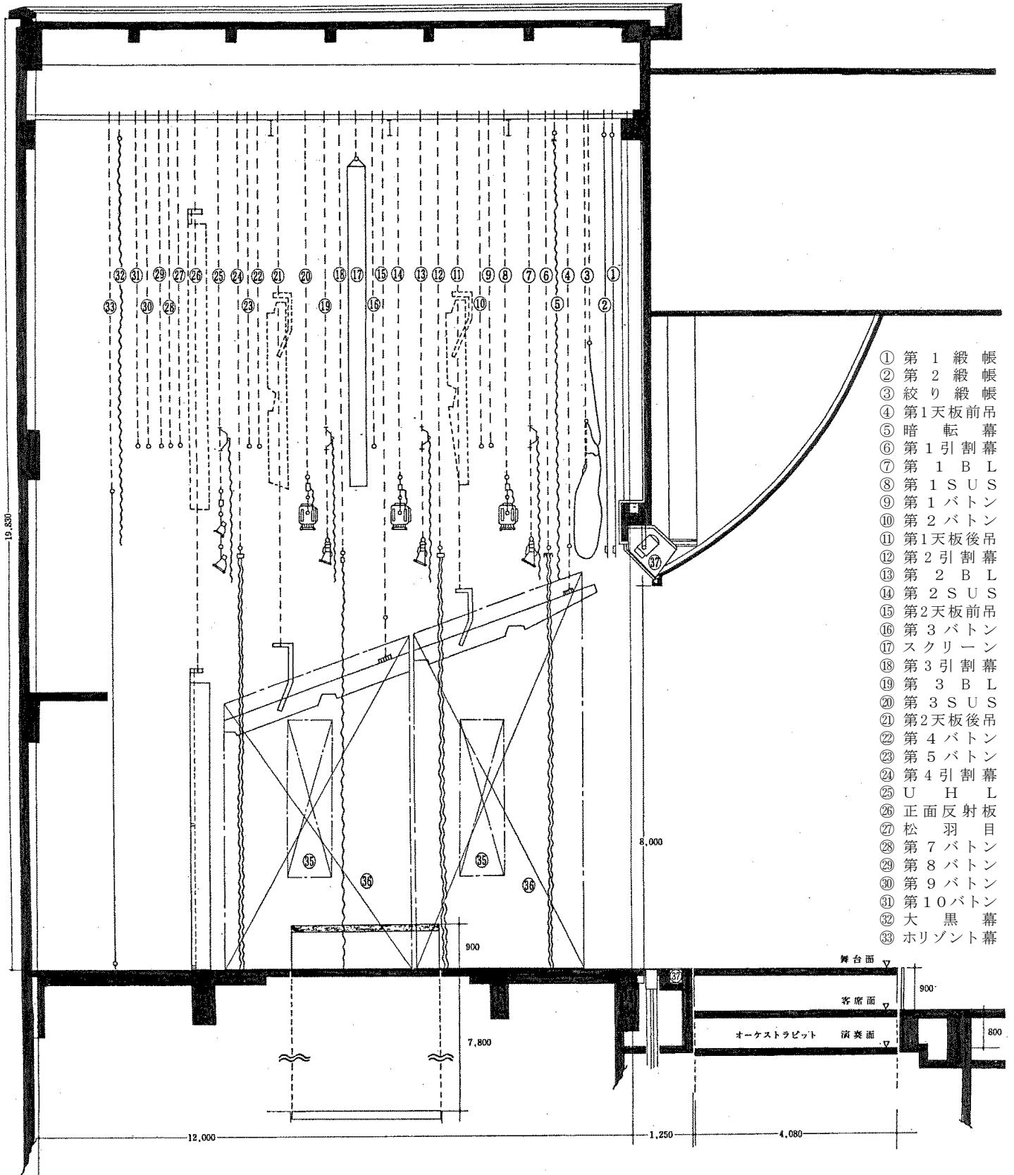
下関市民会館 大ホール舞台断面図
